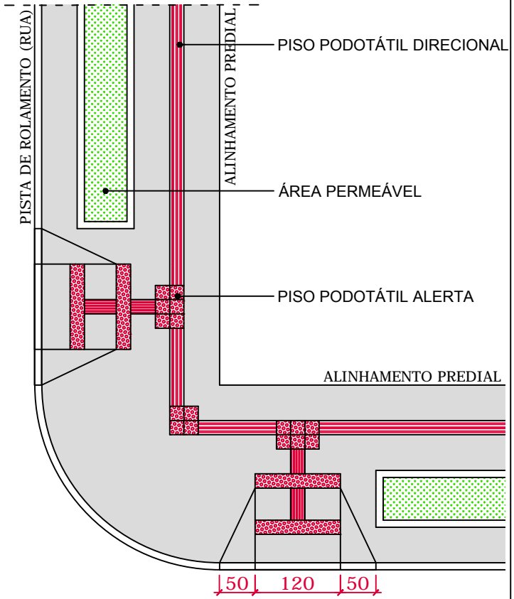
04 | PLANTA-BAIXA: CALÇADAS DE 250 A 500 CM EM ESQUINAS
