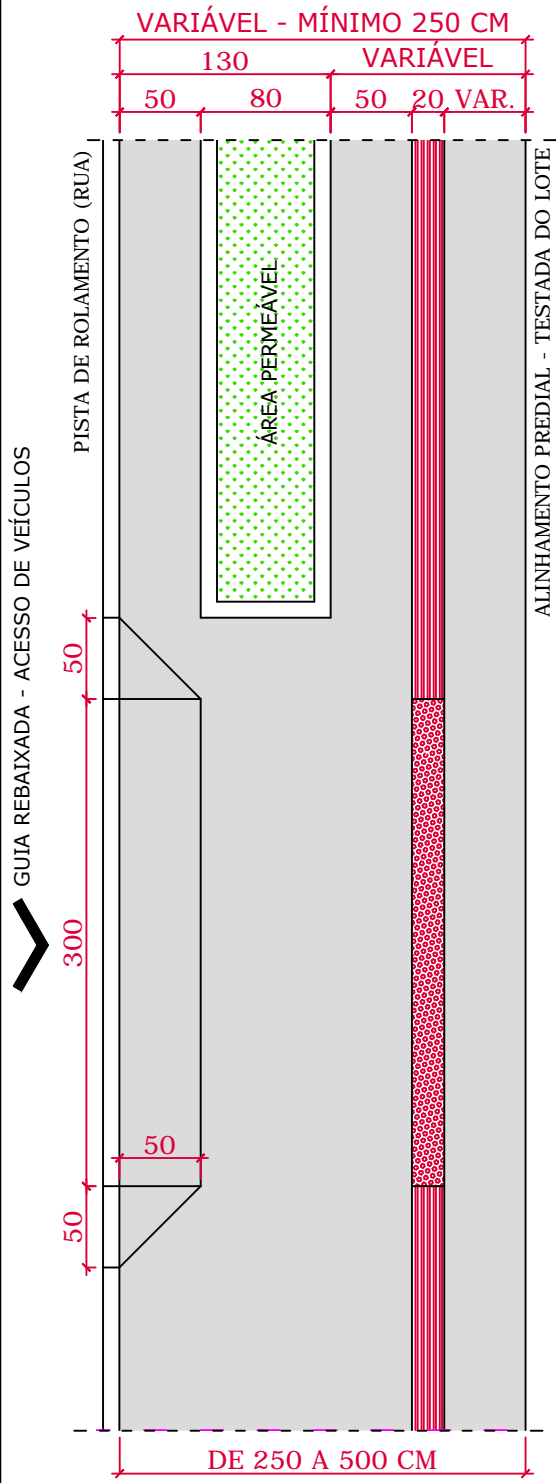
03 | PLANTA-BAIXA: CALÇADAS DE 250 A 500 CM
