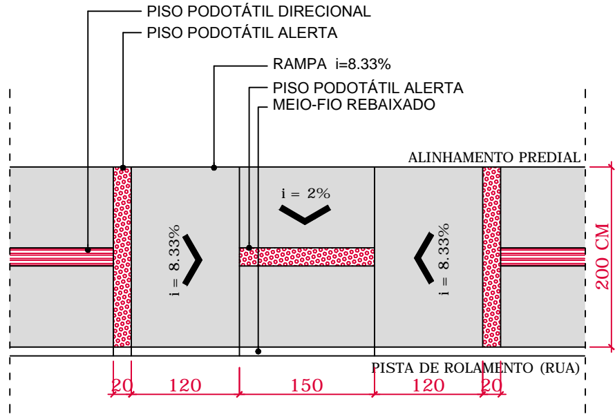
05 | PLANTA-BAIXA: RAMPA CALÇADAS COM 200 CM DE LARGURA
