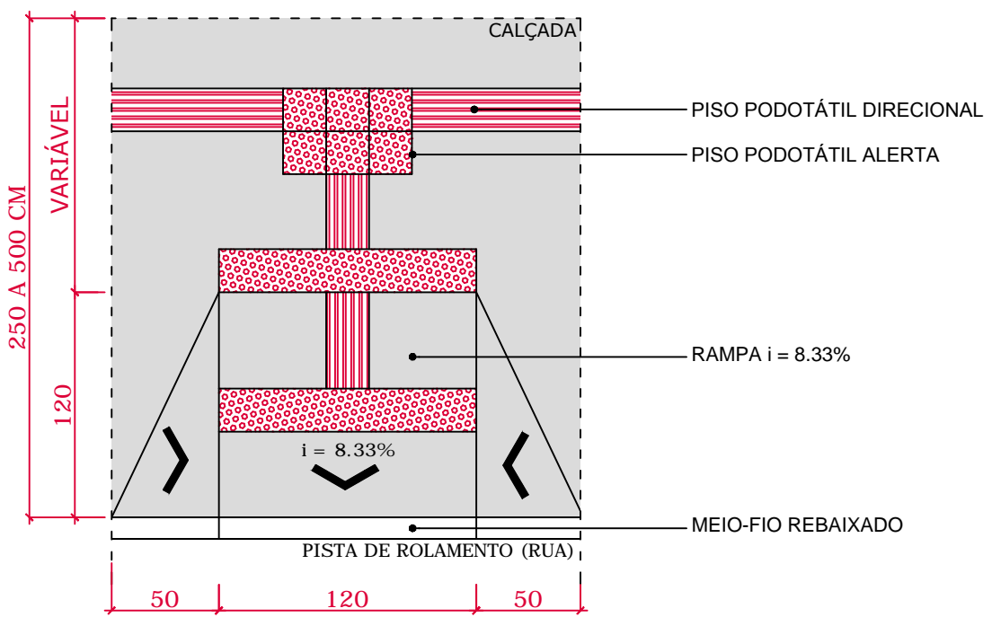
06 | PLANTA-BAIXA: RAMPA CALÇADAS DE 250 A 500 CM DE LARGURA
